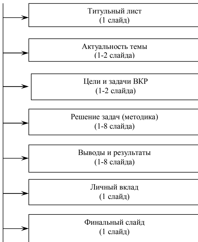
Рис. 4. Структура презентации
